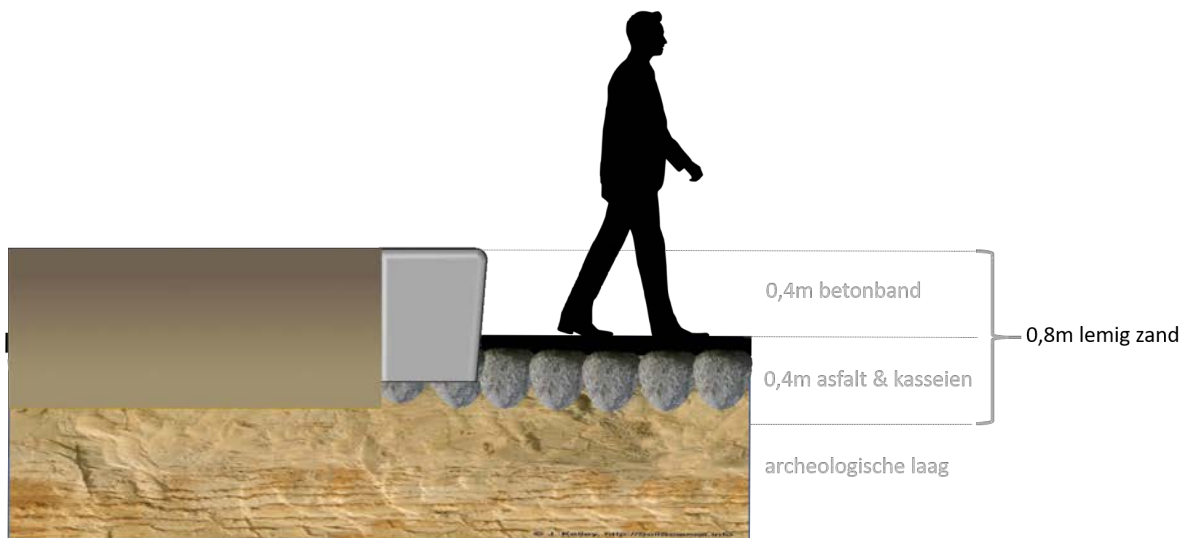
Snede parking – ontwerpprincipe opbouw
